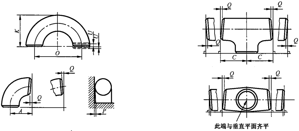
图 14 公差简图
