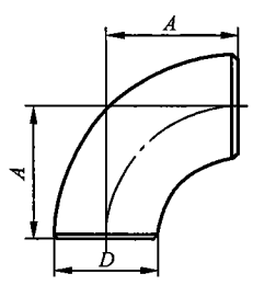
图 4 短半径 90°弯头
