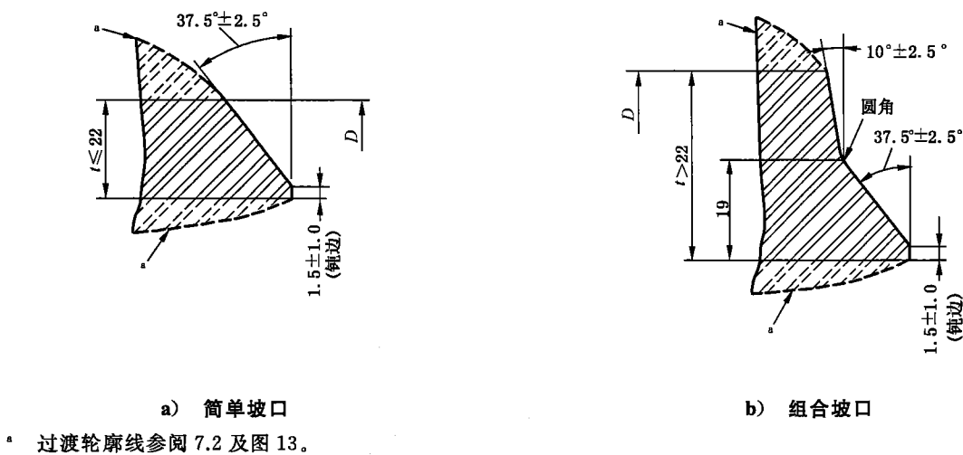
图 12 管件端部坡口形状及尺寸
