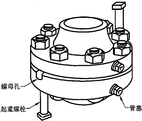
图 A.7.1 带颈对焊孔板法兰结构示意图(径向测压孔)
