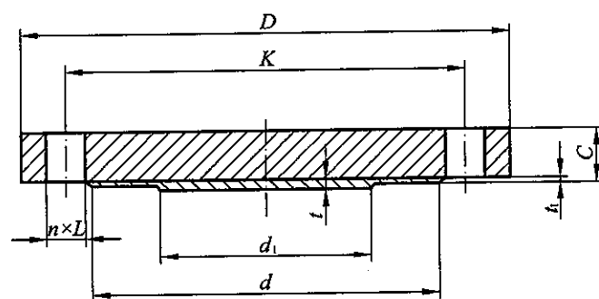
突面 (RF)
