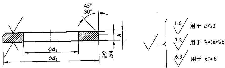
图 A.0.1 平垫圈基本型式 表 A.0.1 紧固件用平垫圈尺寸 (mm)
