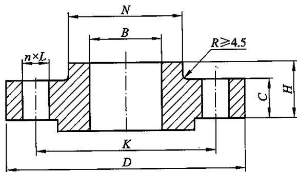
图 B.6.2-1 带颈平焊夹套法兰
