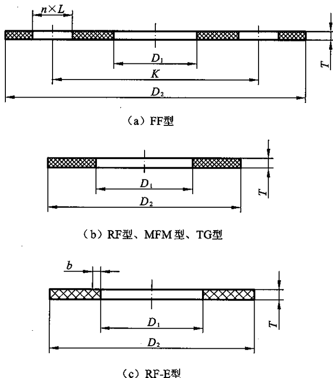
图 4.0.1 垫片的型式
