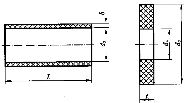
图 B.0.2 绝缘衬套和绝缘垫圈
