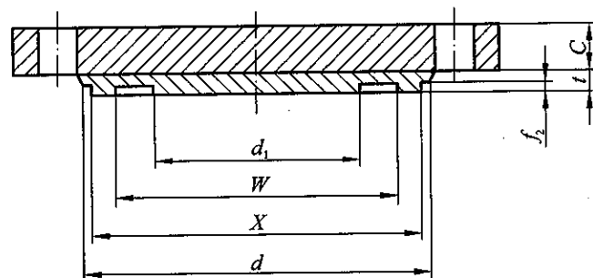
榫面 (T)
