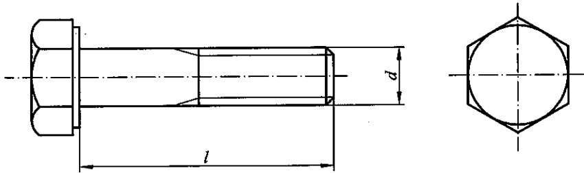
图 3.2.1 六角头螺栓
