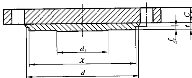
凸面 (M)
