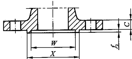
榫面 (T)
